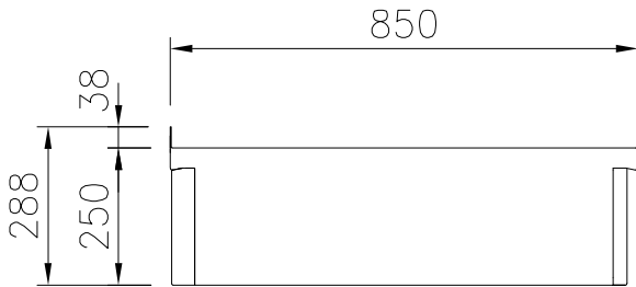
Zij aanzicht
